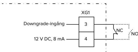
Fig. 16: Principkopplingsschema: anslutning av en extern brytarkontakt (standardinställning: NO)
