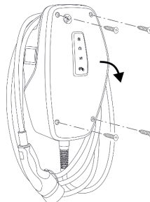
Kuva 5: Tuotteen avaaminen
