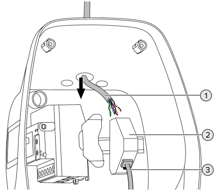
Kuva 14: Tietojohdon liittäminen (esimerkki)
