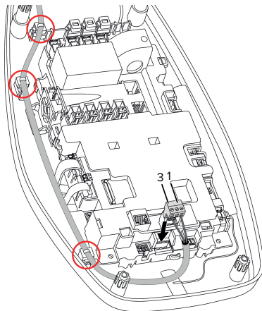
Kuva 9: Työvirtalaukaisijan liitäntä
