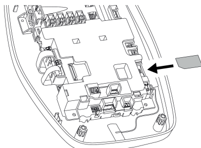
Fig. 11: Isætning af SIM-kort
