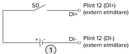
Fig. 17: Styrning via ett kopplingsrelä och ytterligare en spänningsförsörjning (vid leveranstillstånd)
