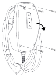
Fig. 5 : Ouverture du produit
