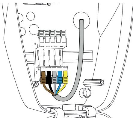
Kuva 8: Jännitesyötön liitäntä (esimerkki)
