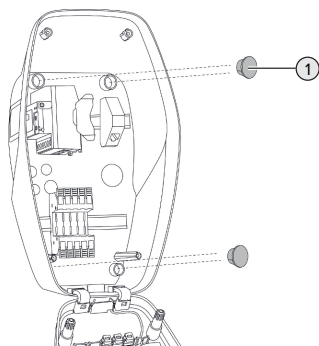
Kuva 7: Sulkutulpat
