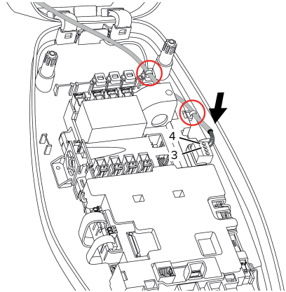
Kuva 15: Downgrade-tulon liitäntä
