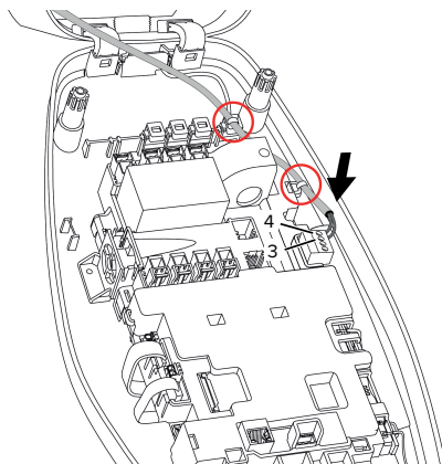
Fig. 15: Tilslutning downgrade-indgang
