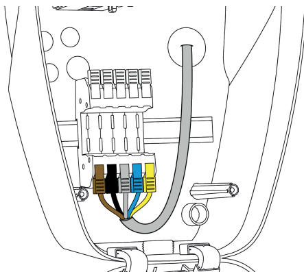
Fig. 8: Anslutning matarspänning (exempel)
