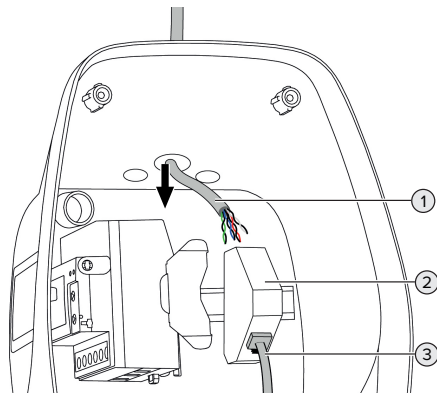
Fig. 14: Anslut dataledning (exempel)
