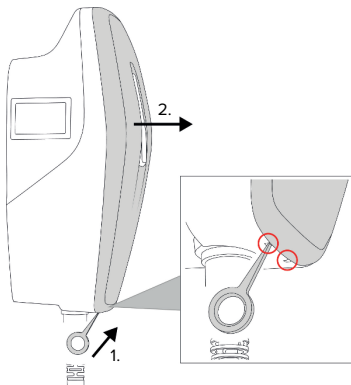
Kuva 4: Front Coverin irrottaminen
