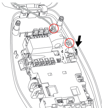
Abb. 15: Anschluss Downgrade-Eingang
