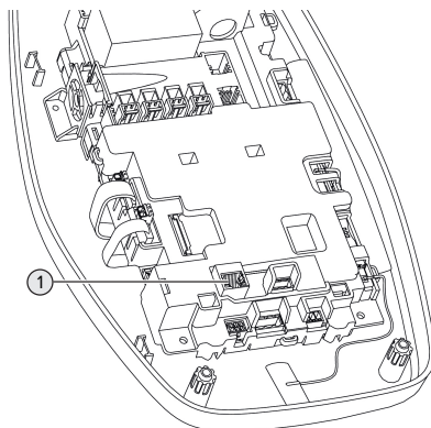
Fig. 13: Ethernet-anslutning
