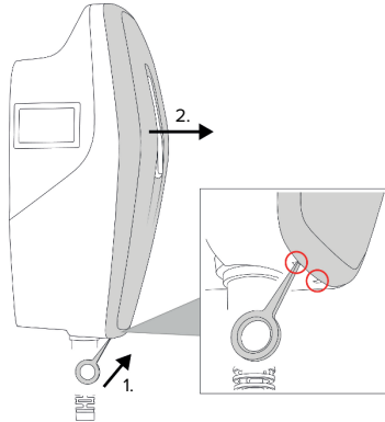
Fig. 4: Lossa frontkåpan
