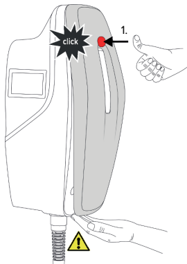
Kuva 20: Front Coverin kiinnitys – 1
