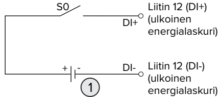
Kuva 17: Ohjaus kytkentäreleellä ja ylimääräisellä jännitesyötöllä (toimitustilassa)
