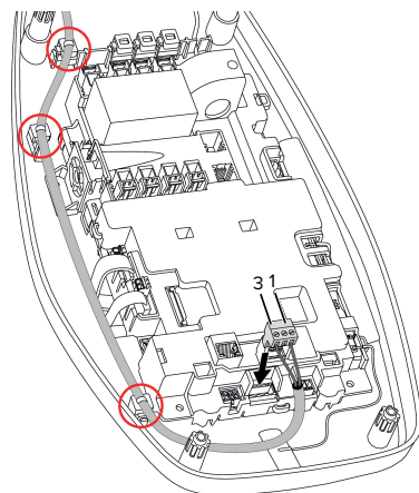
Fig. 9: Tilkobling arbejdsstrømsudløser
