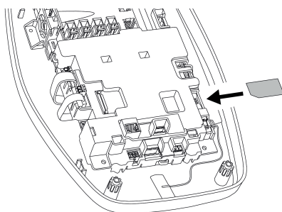
Fig. 11: Sätta i SIM-kort
