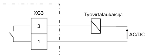
Kuva 10: Periaatekytkentäkaavio: ulkoisen työvirran laukaisijan liitäntä
