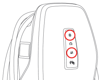
Fig. 12: Aktivering af Access Point
