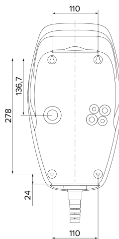
Fig. 6 : Dimensions de perçage [mm]
