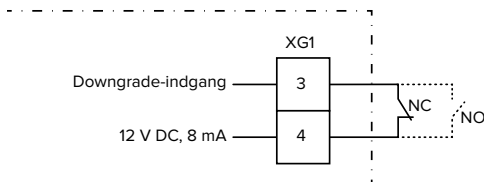
Fig. 16: Principskema: tilslutning af en ekstern omskifterkontakt (standardindstilling: NO)
