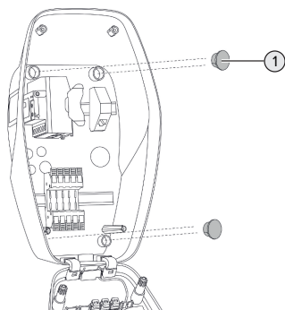
Fig. 7: Täcklock
