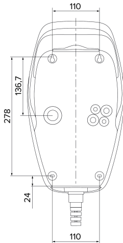
Fig. 6: Bormått [mm]
