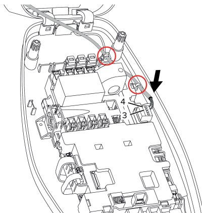
Fig. 15: Anslutning av downgrade-ingång
