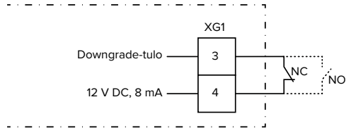
Kuva 16: PeriaatekytKentäkaavio: ulkoisen kytKentäkontaktin liitäntä (vakioasetus: NO)
