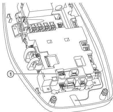
Abb. 13: Ethernet-Anschluss
