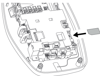
Kuva 11: SIM-kortin asettaminen
