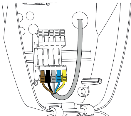
Fig. 8: Tilslutning strømforsyning (eksempel)
