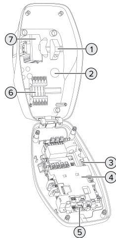
Afb. 3: Binnenaanzicht
