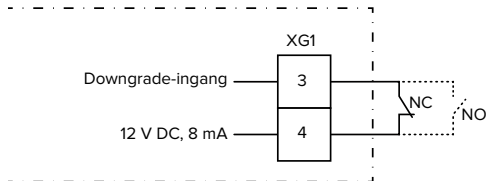
Afb. 16: Principeschema: aansluiting van een extern schakelcontact (standaardinstelling: NO)
