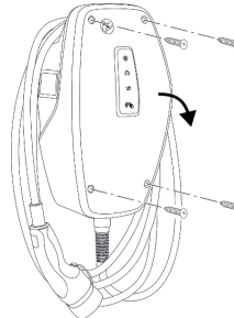
Fig. 5: Öppna produkten
