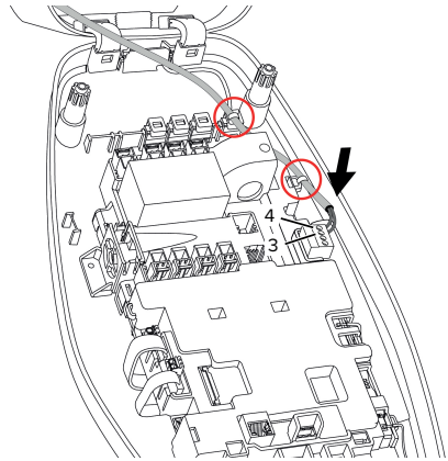
Afb. 15: Aansluiting downgrade-ingang
