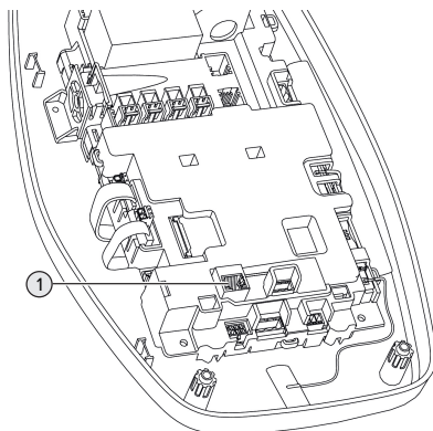
Kuva 13: Ethernet-liitäntä
