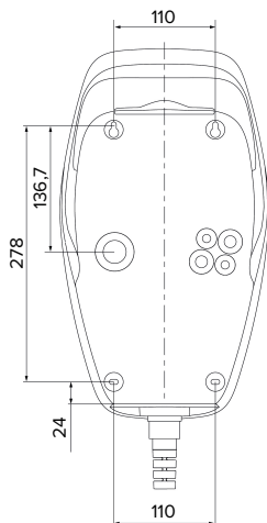
Kuva 6: Porausmitat [mm]
