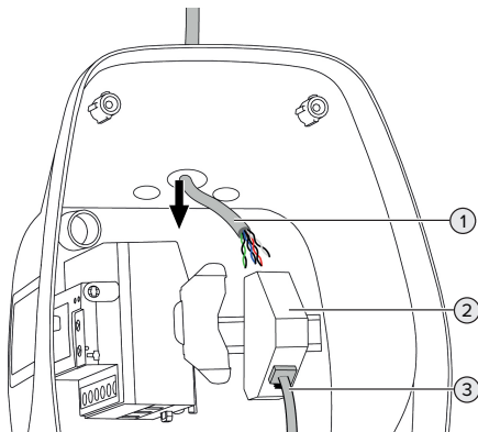
Fig. 14: Tilslutte netværkskablet (eksempel)
